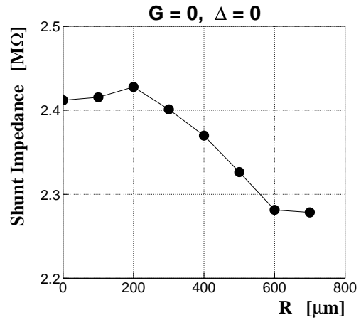
図8: R 面取りサイズの関数としてのシャント・インピーダンス( G = \Delta = 0 の場合)。
