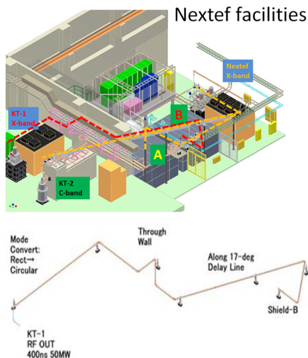
図 1: Nextef 高電界試験施設 (上図) と、新設したシールド B への大電力高周波移送ライン (下図)。
